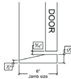
Jamb size
